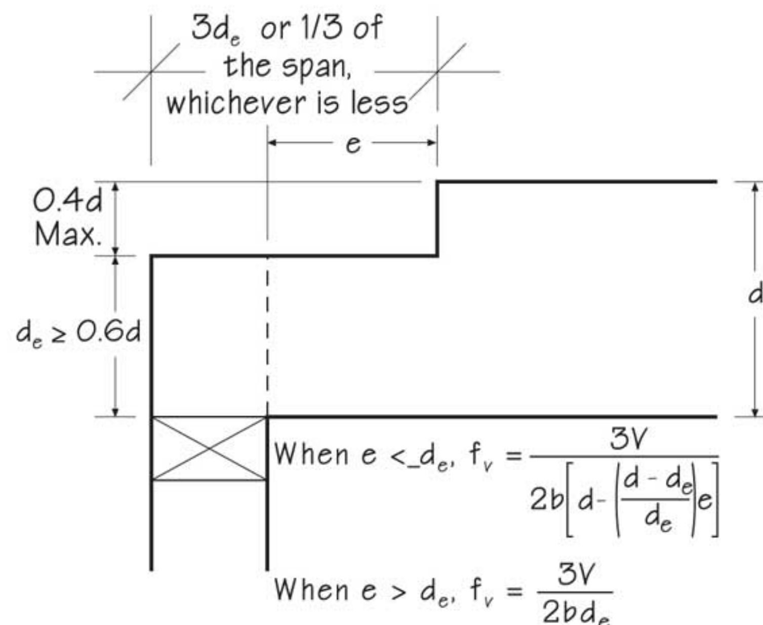
(d) Compression-side Notch
