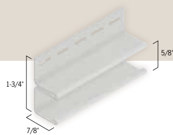
F Trim (1178)
